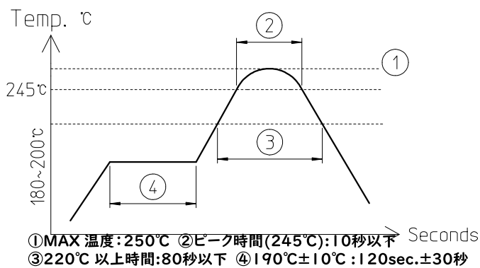
付図 2. リフロープロファイル
